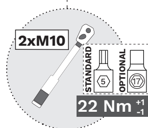
AVENTO 3
